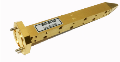
Fig 1 THZWGP-05-100 140-220 GHz
