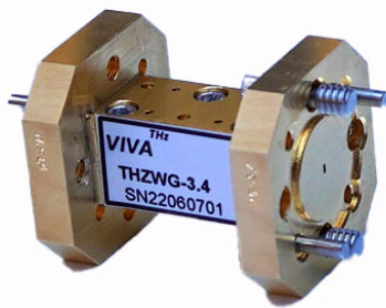
Fig 3 Model THZWG-3.4
