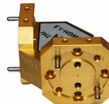
THZWGE-1.5 90 deg H Plane Bend (500-750 GHz) Precision UG387/U-M w/IEEE 1785.2 flange
