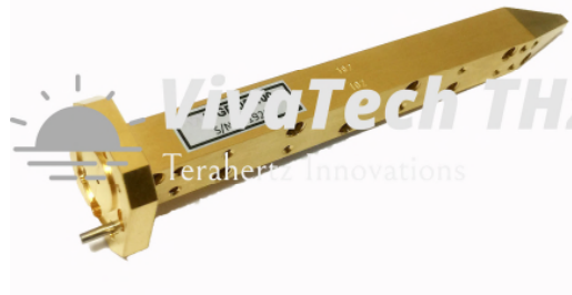
Fig 1 THZWGP-05-100 140-220 GHz
