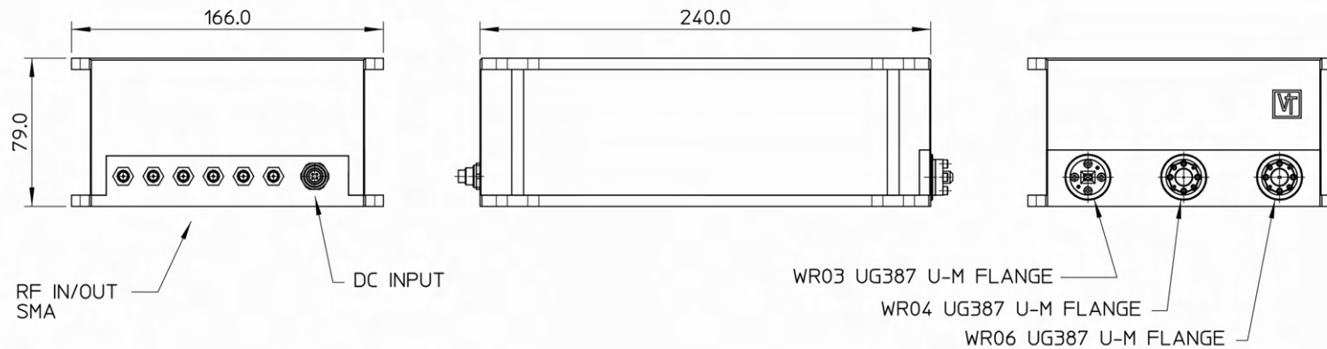
Fig 5 110-330 GHz Converter Module
