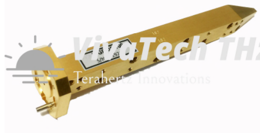
Fig 1 THZWGP-05-100 140-220 GHz
